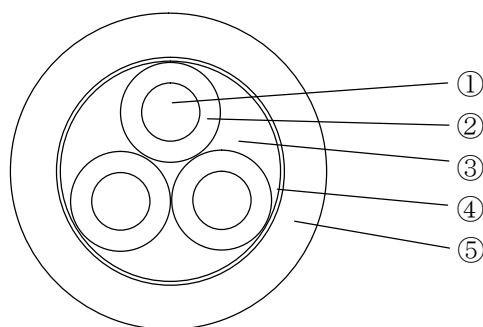
断面図（例：3心）
