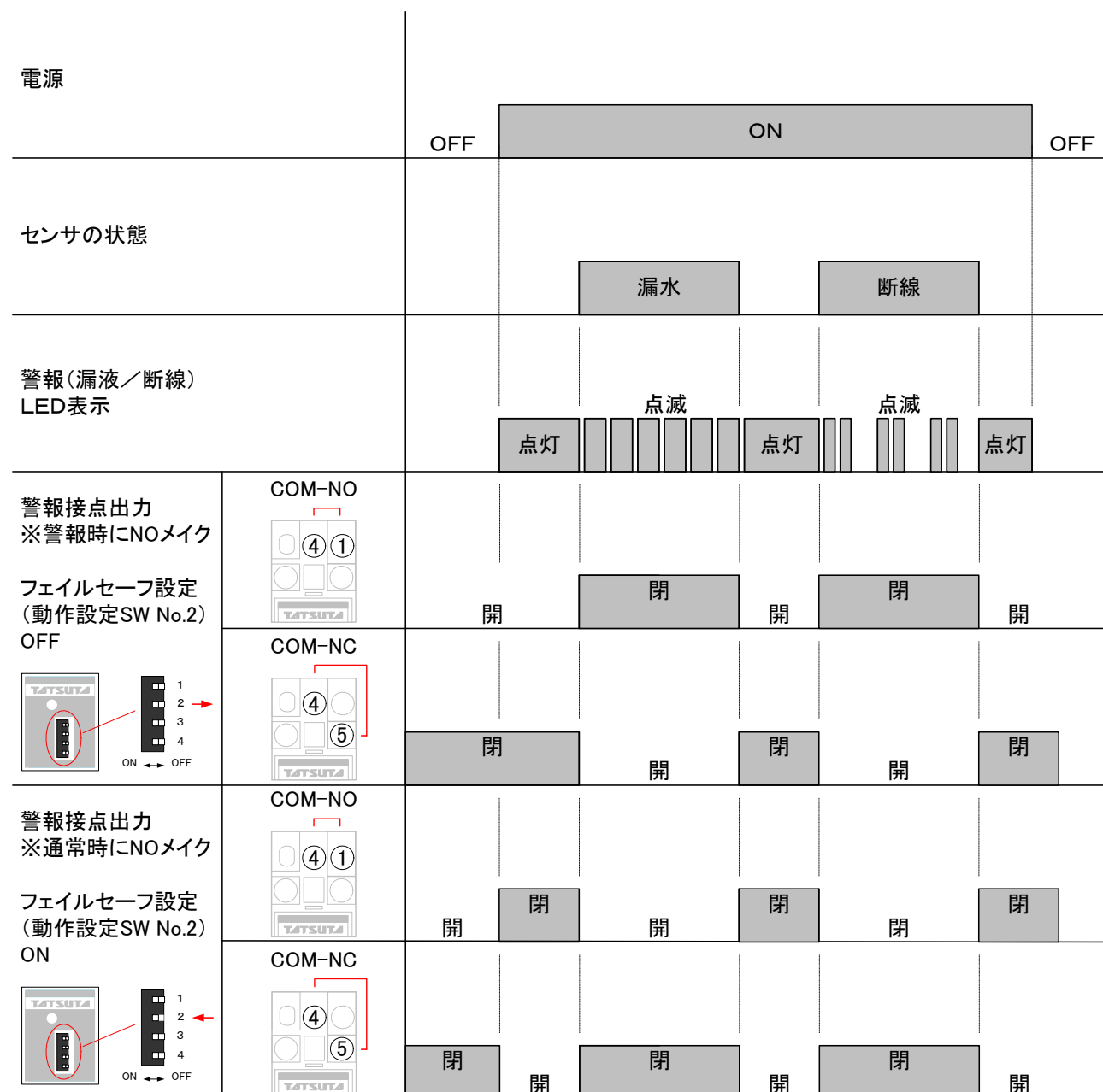
図 2. 動作チャート
