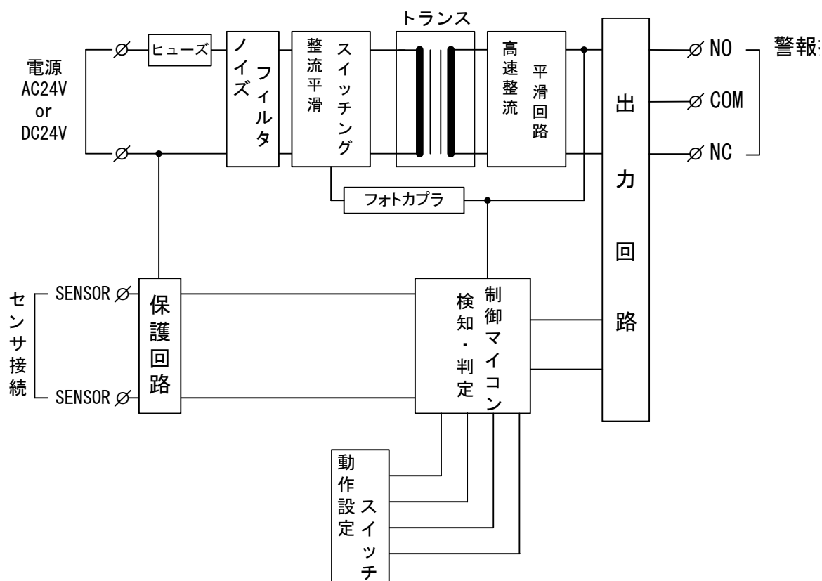
図 1. 検知器の内部構成
