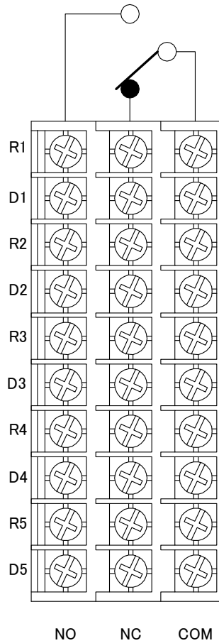
図－5. 個別制御出力接点
