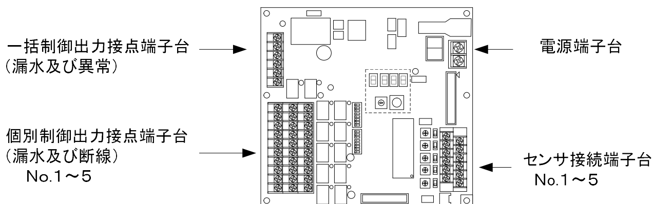
図-1. 端子台配置図
