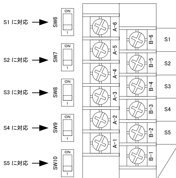
図-3. センサ端子台
