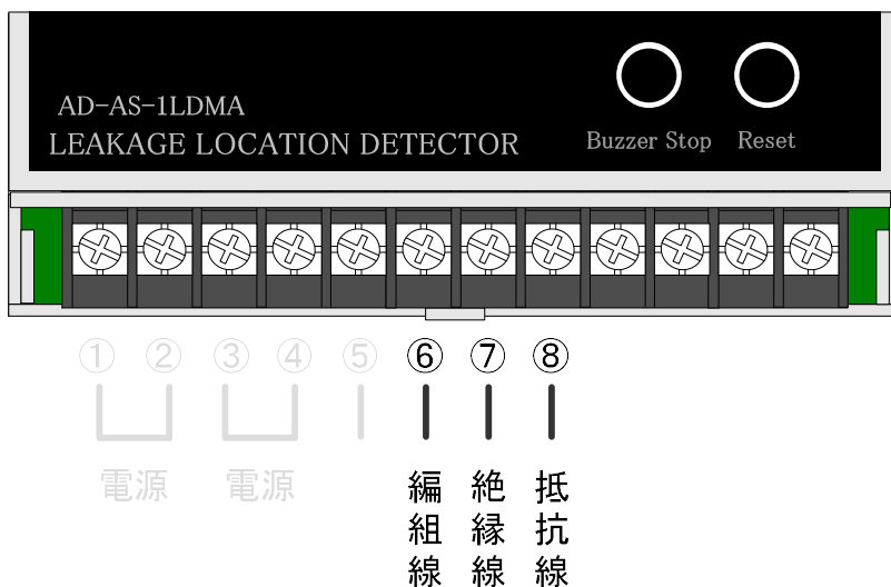
図-5. センサ接続端子台
