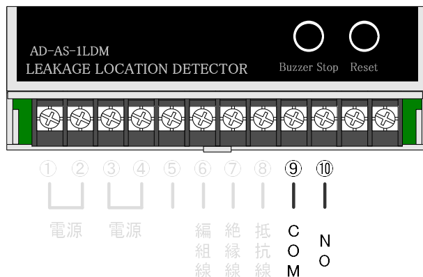
図一6. 制御出力接点
