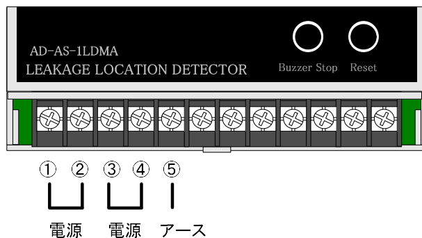
図-3. 端子台配置図
