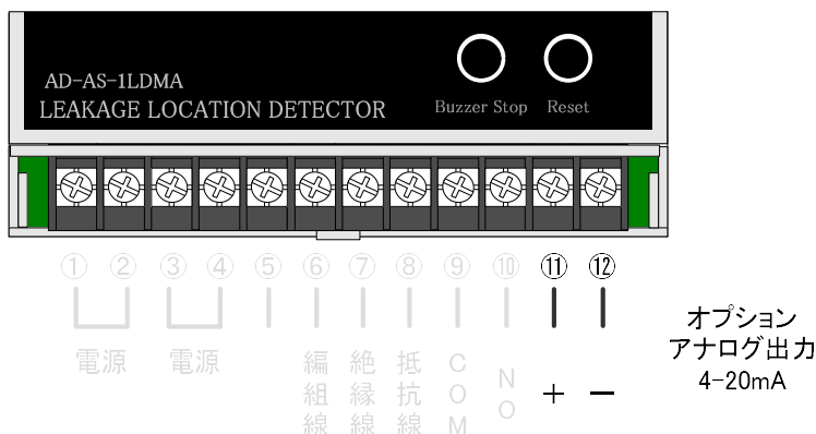
図-7. 漏水位置データ出力の接続
