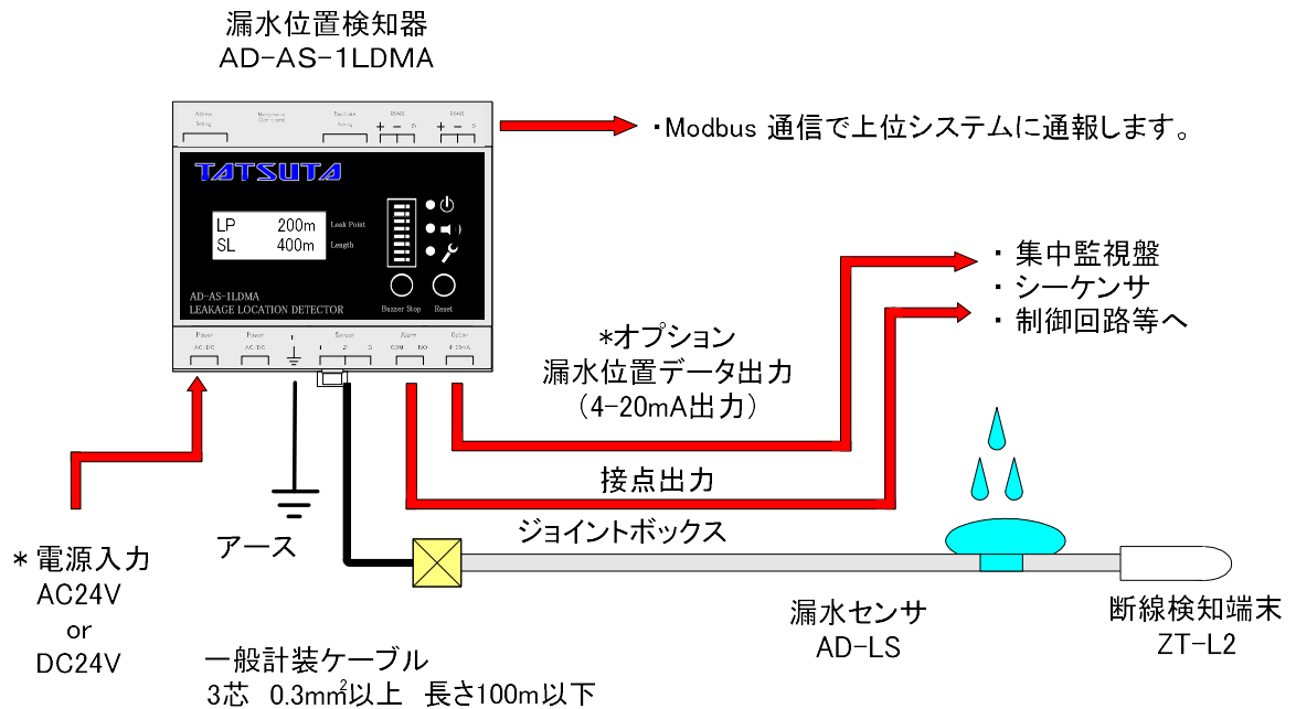
図-2. 漏水位置検知システム
