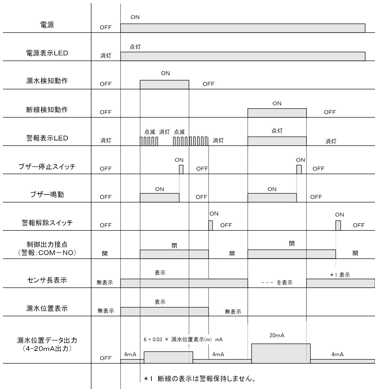
図-14. 動作チャート2
