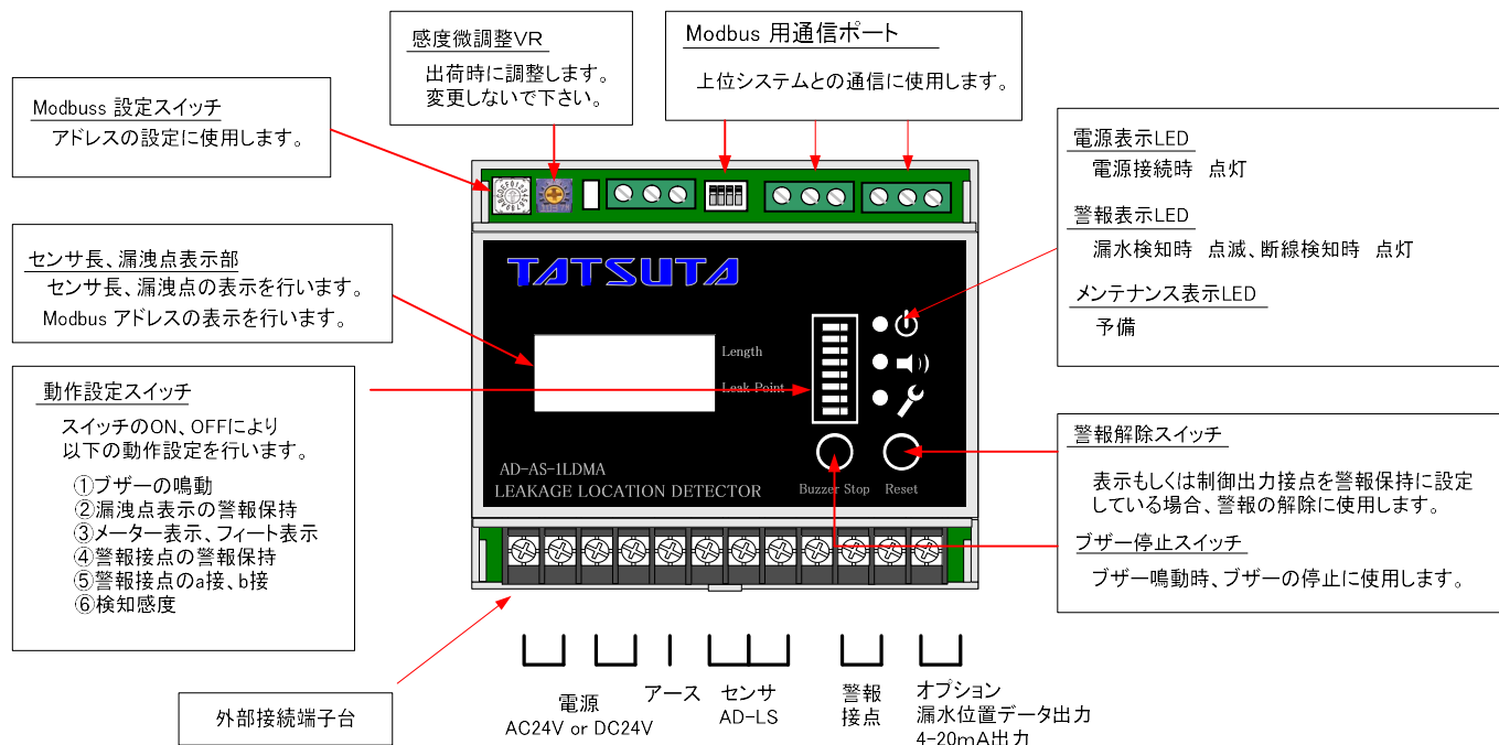
図-1. 漏水位置検知器各部説明
