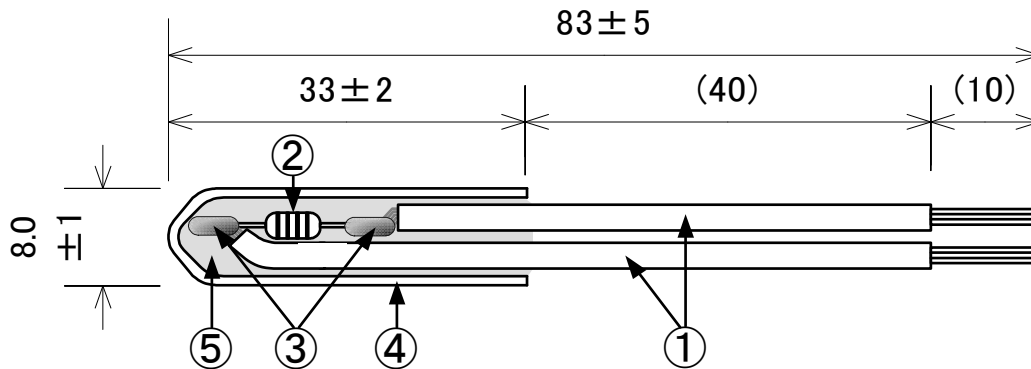
図-1. ZT-SR姿図(キャップ部断面)
