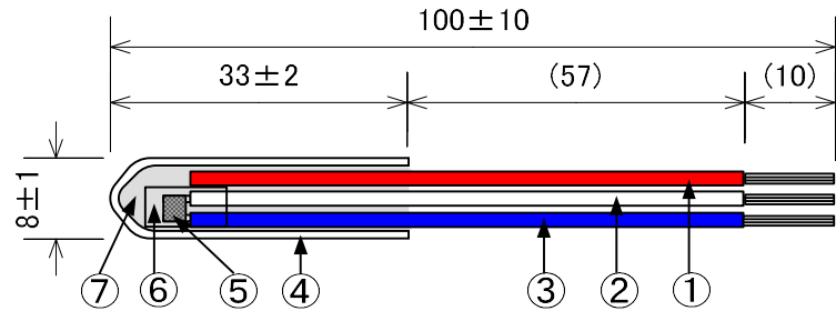
図-1. ZT-L2姿図(キャップ部断面)
