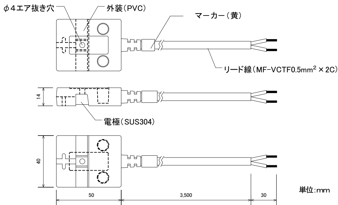
図-1. AD-PA-Nセンサ姿図
