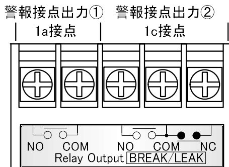
図 2 警報接点出力の出力端子
