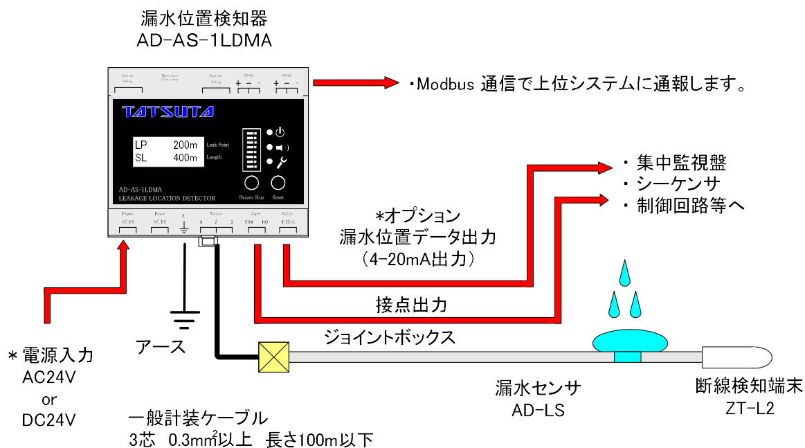
図一1. 漏水位置検知システム
