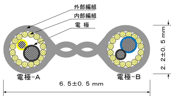
図－2 AD-BFL センサ断面図
