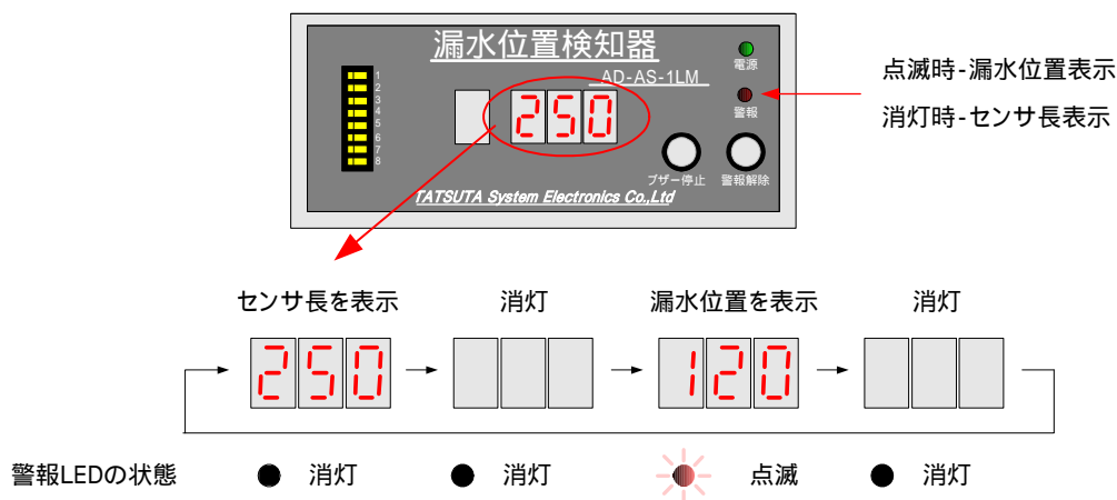
図-11. 漏水検知時の表示
