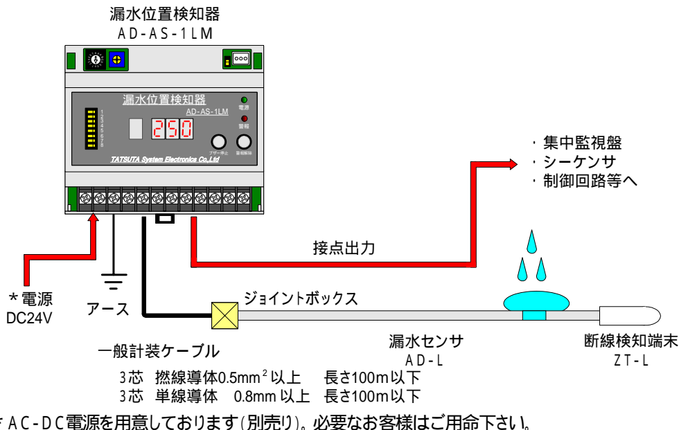
図 - 2. 漏水位置検知システム
