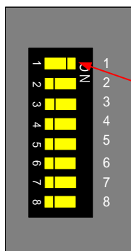
図-13. ブザー設定
