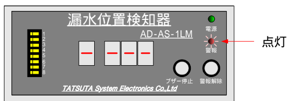
図-10 断線検知時の表示
