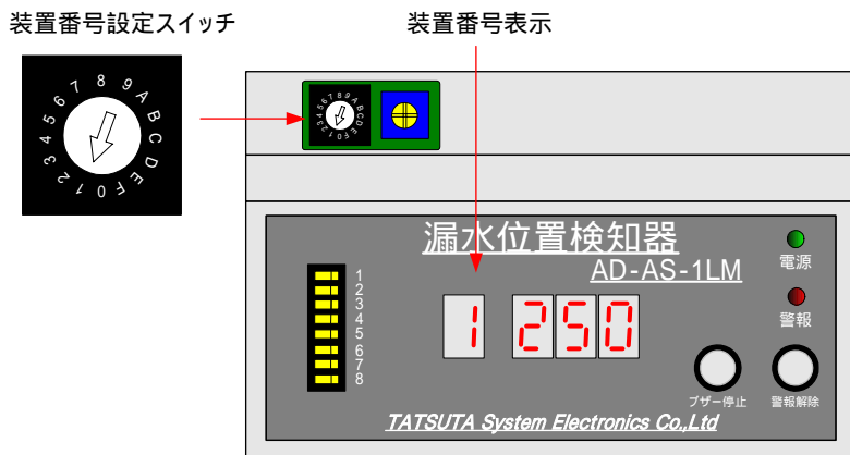
図 - 16 . 装置番号表示
