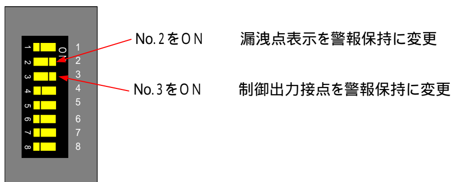
図 - 14. 警報保持の設定
