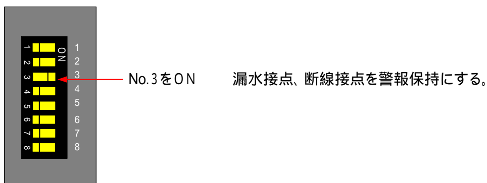
図 - 8 . 漏水・断線接点の警報保持設定
