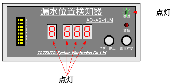
図-9. 電源立上げ時の動作
