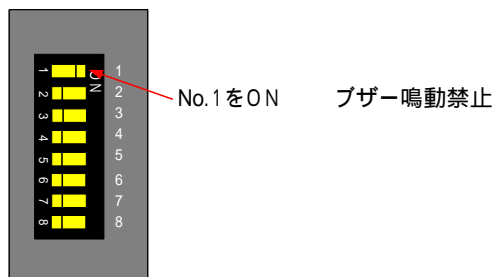
図 - 18. ブザー設定
