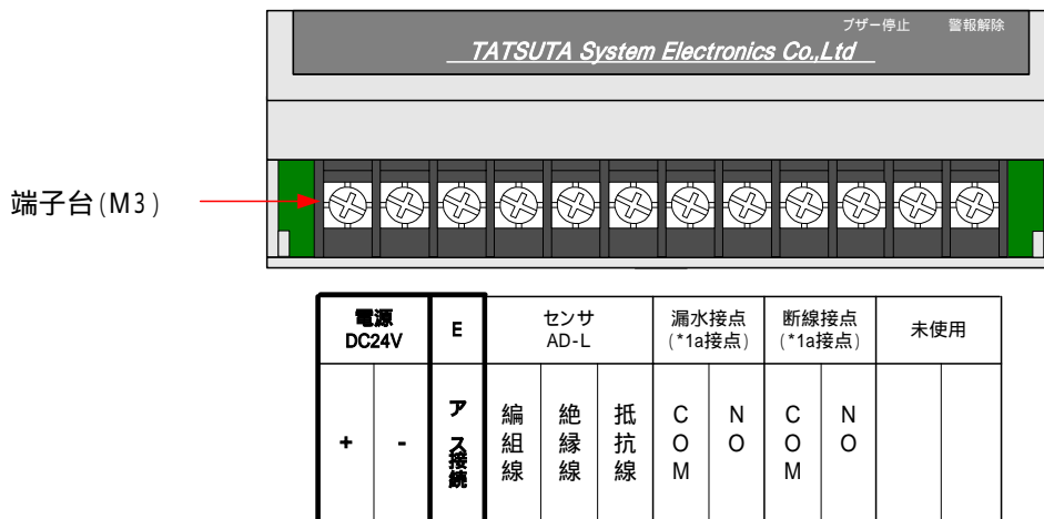
図 - 3. 端子台配置図
