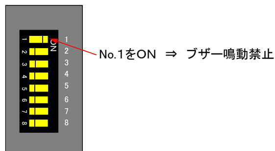
図-16. ブザー設定
