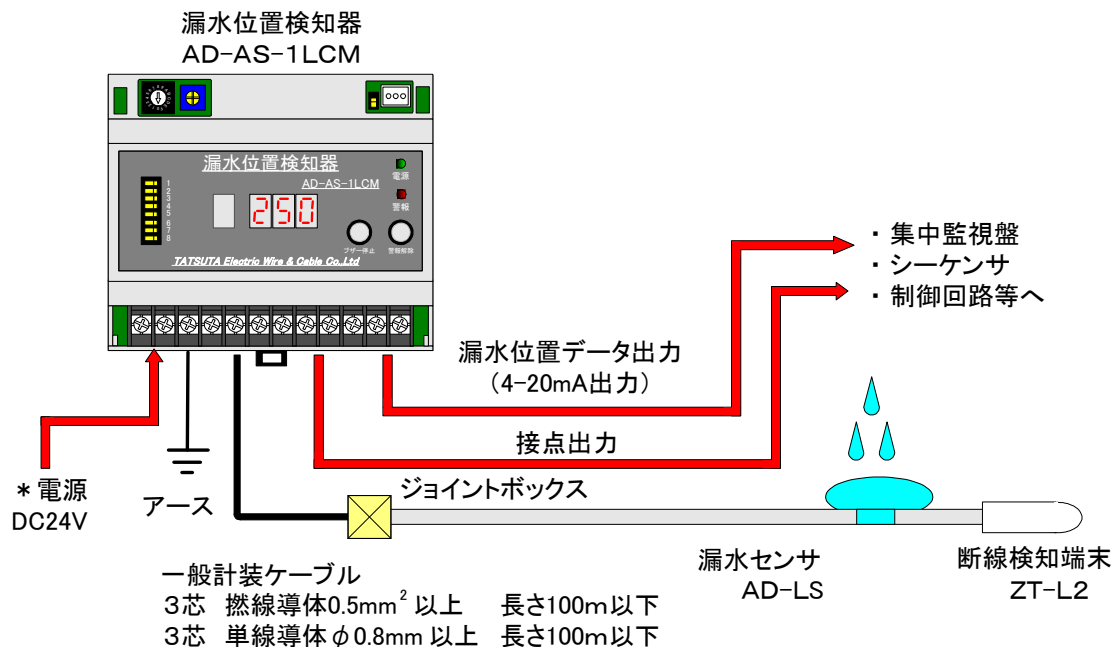
図-2. 漏水位置検知システム
