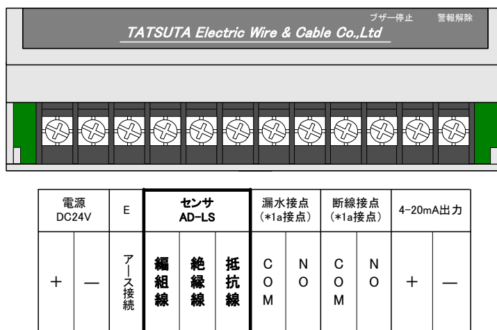
図-3. 端子台配置図
