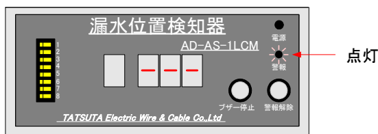
図-13断線検知時の表示
