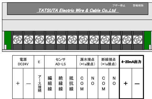
図-9. 漏水位置データ出力の接続
