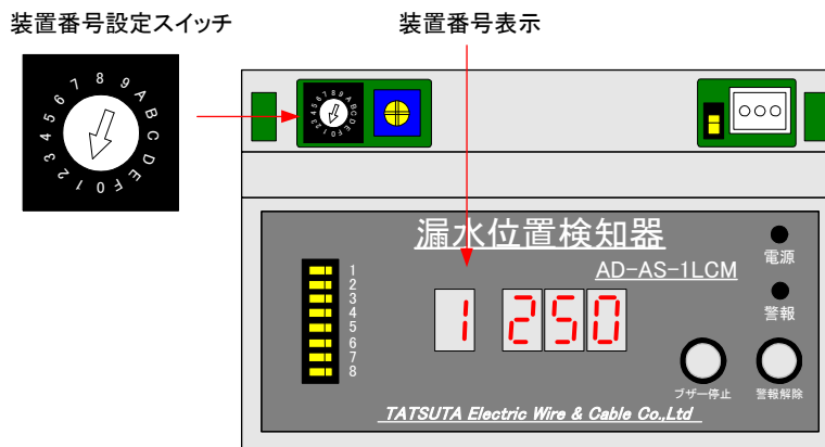
図－19. 装置番号表示
