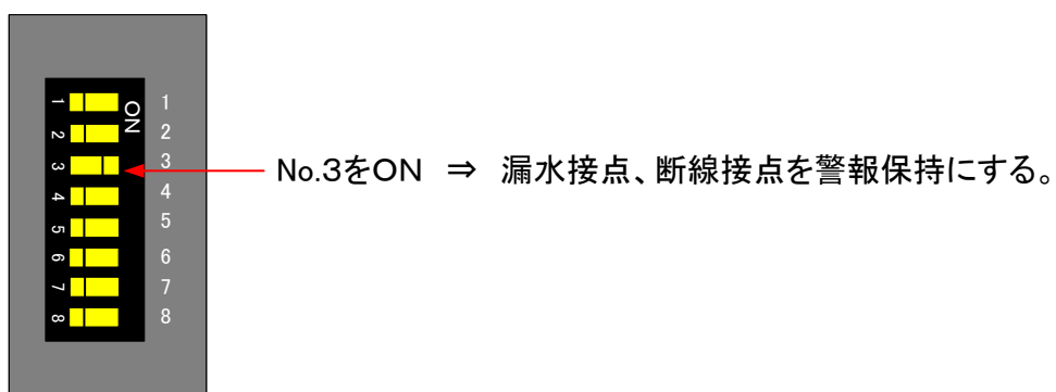
図-8. 漏水・断線接点の警報保持設定
