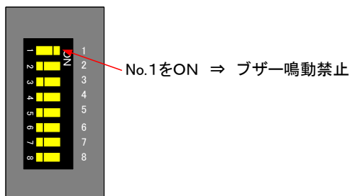
図-21. ブザー設定
