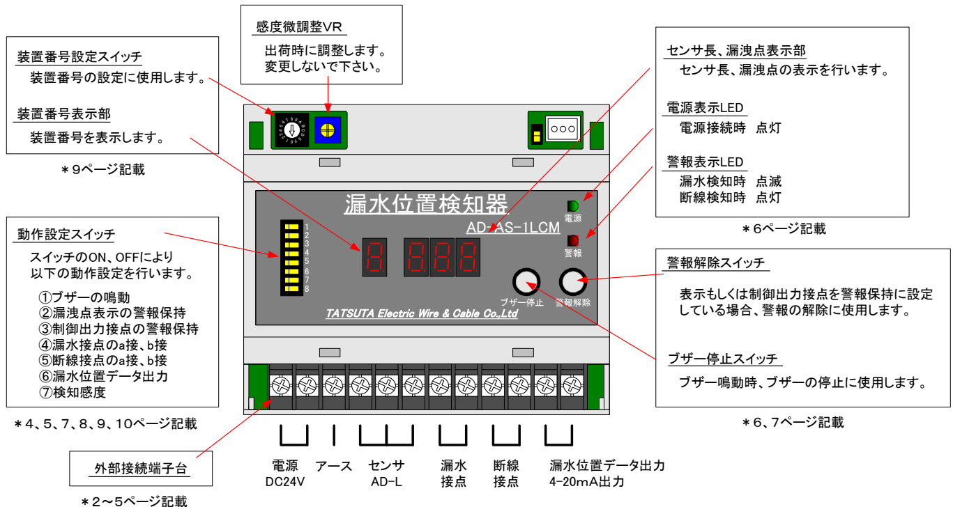
図-1. 漏水位置検知器各部説明
