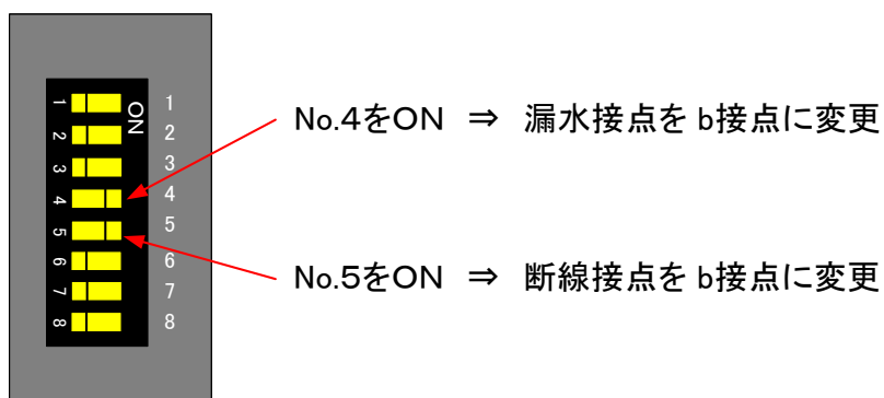
図-7. 漏水・断線接点動作設定
