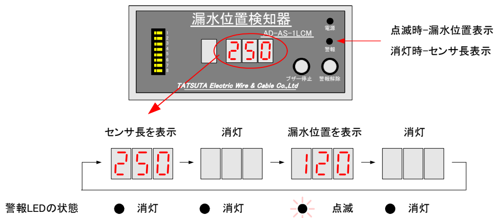
図-14. 漏水検知時の表示
