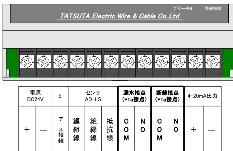
図-6. 制御出力接点
