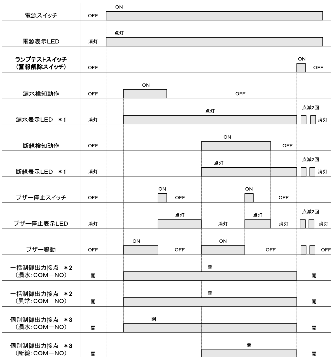
図-3. 動作チャート2
