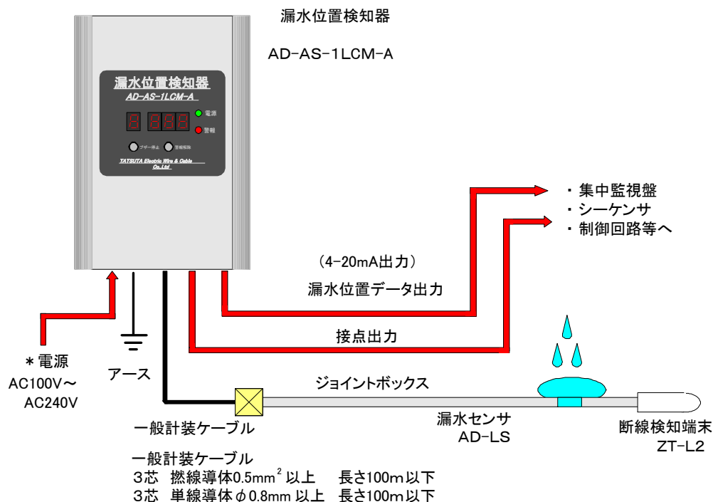
図-2. 漏水位置検知システム
