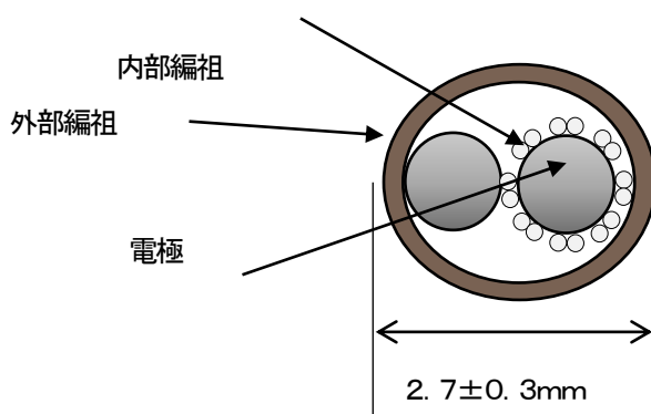
図-2. 断面図
