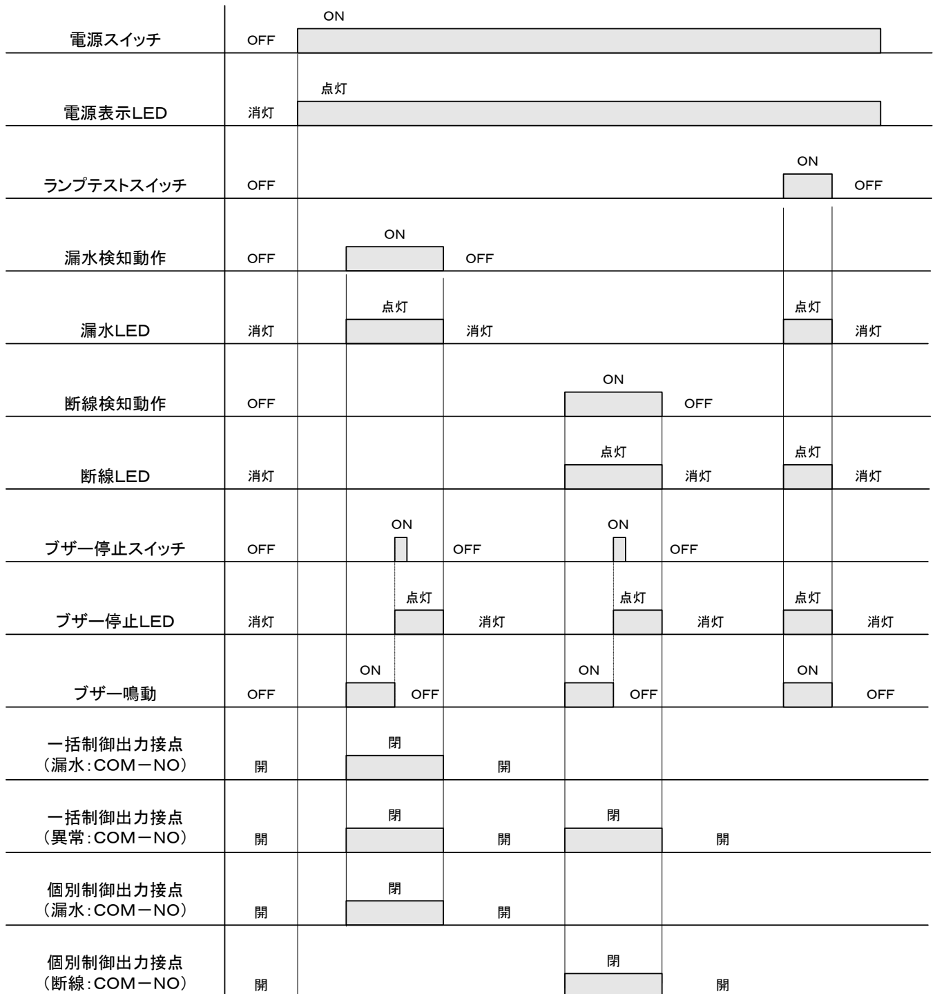
図-7. 動作チャート1
