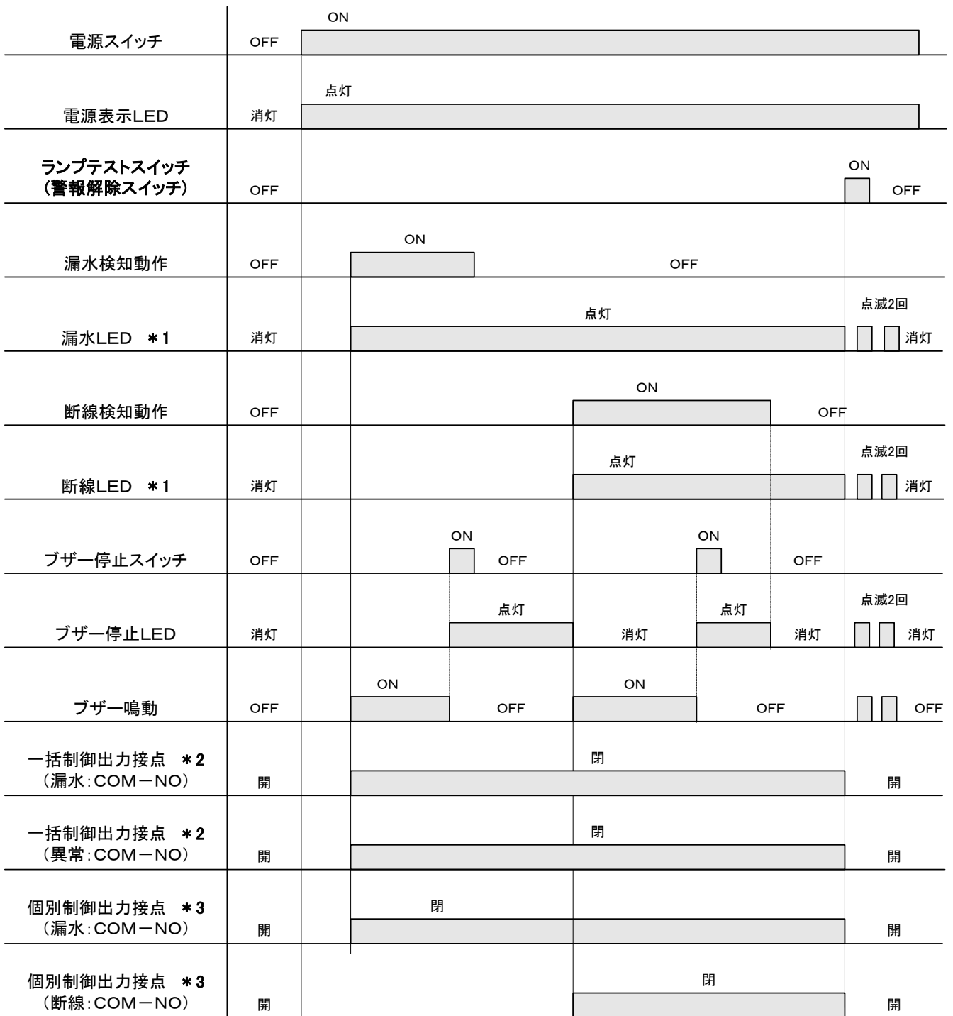
図-8. 動作チャート2
