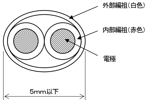
図-2. AD-Rセンサ断面図
