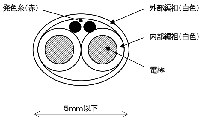
図-2. AD-Hセンサ断面図
