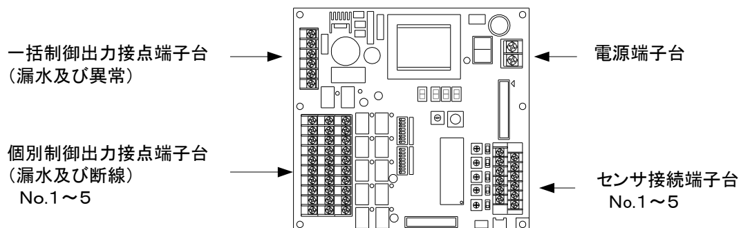
図-1. 端子台配置図
