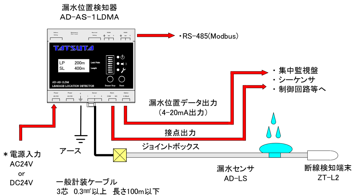
図-1.漏水位置検知システム
