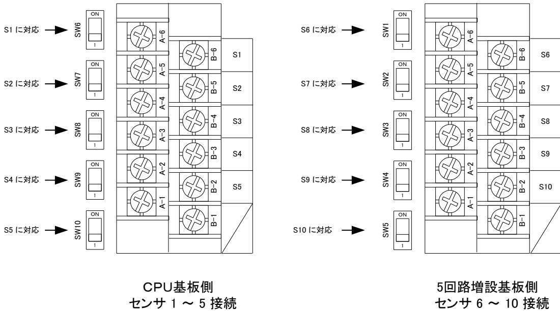
図-3. センサ端子台
